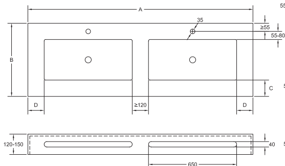
*Dimensions pour siphon Quare
